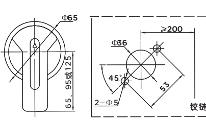
圆形延伸旋转手柄开孔尺寸图
