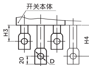
RDM5L-400、800板后接线
